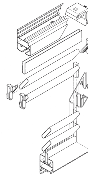
Lama Fija
