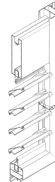
Lama Móvil
